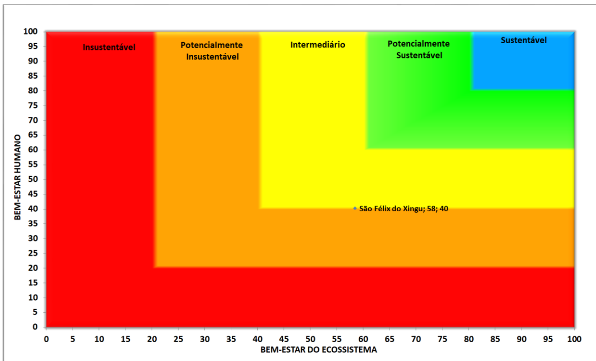
Figura 4 — Gráfico bidimensional do Barômetro da Sustentabilidade do município de São Félix do Xingu.
